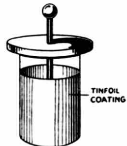
Fig. 13. The Complete Leyden Jar
